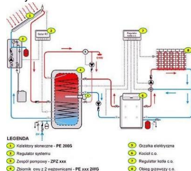
PRZYKŁADOWY SCHEMAT BUDOWY INSTALACJI SŁONECZNEJ DO PODGRZEWANIA CIEPŁEJ WODY UŻYTKOWEJ
